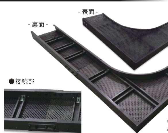
本体とLLを接続
